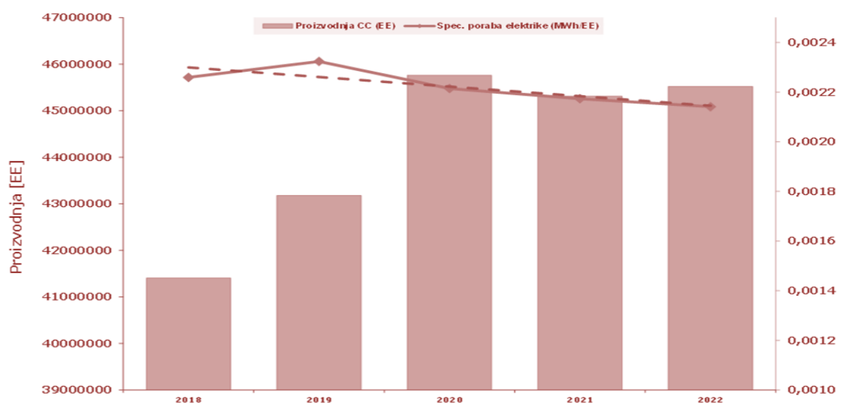
Graf: Specifična poraba električne energije za proizvodnjo na ekvivalentno enoto (EE) v letih 2018–2022 Specifična poraba elektrike za proizvodnjo EE med leti 2018 in 2022
