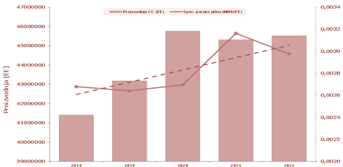
Graf: Specifična poraba zemeljskega plina za proizvodnjo na ekvivalentno enoto (EE) v letih 2018–2022 Specifična poraba plina za proizvodnjo EE med leti 2018 in 2022
