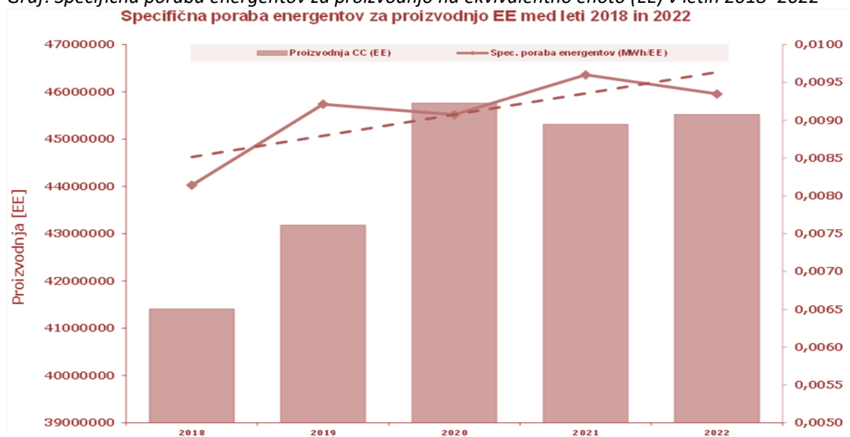
Graf: Specifična poraba energentov za proizvodnjo na ekvivalentno enoto (EE) v letih 2018–2022
