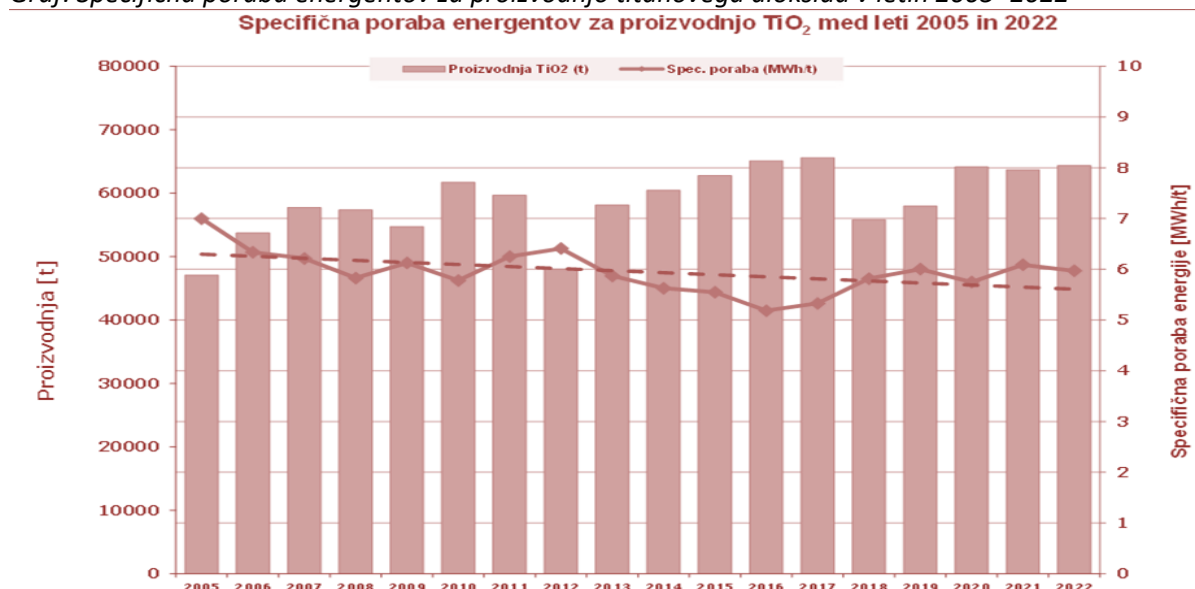
Graf: Specifična poraba energentov za proizvodnjo titanovega dioksida v letih 2005–2022
